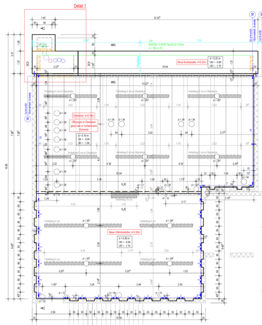
Schalung Decke über Technik
